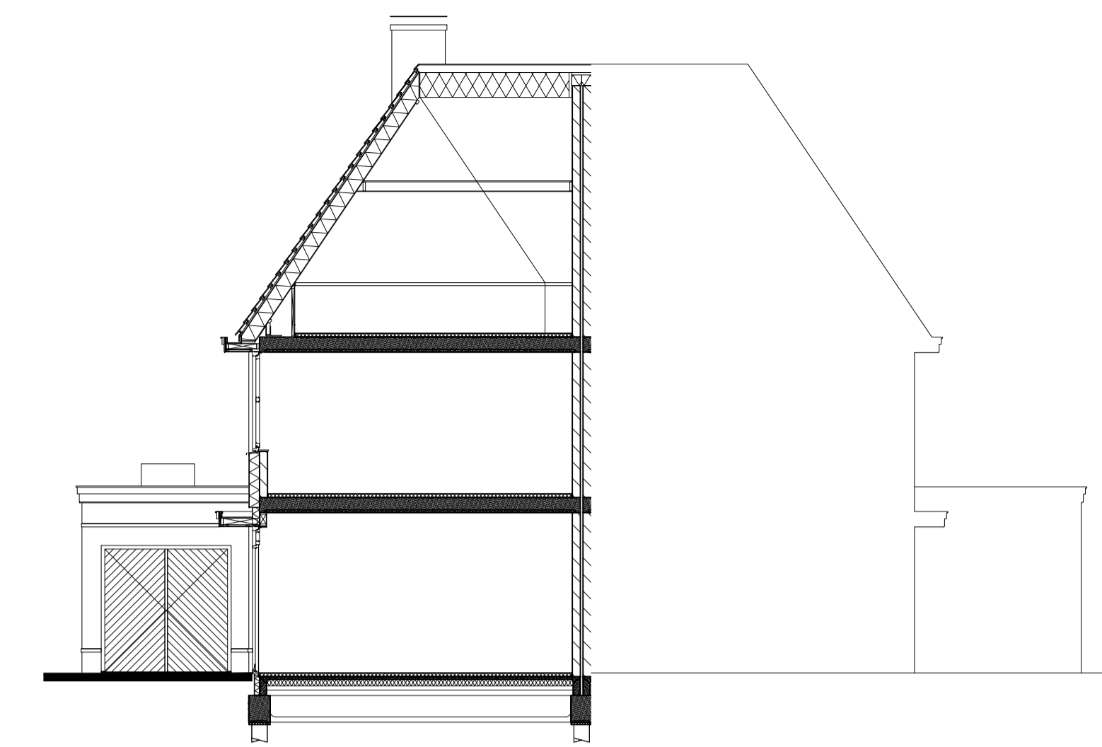
doorsnede
