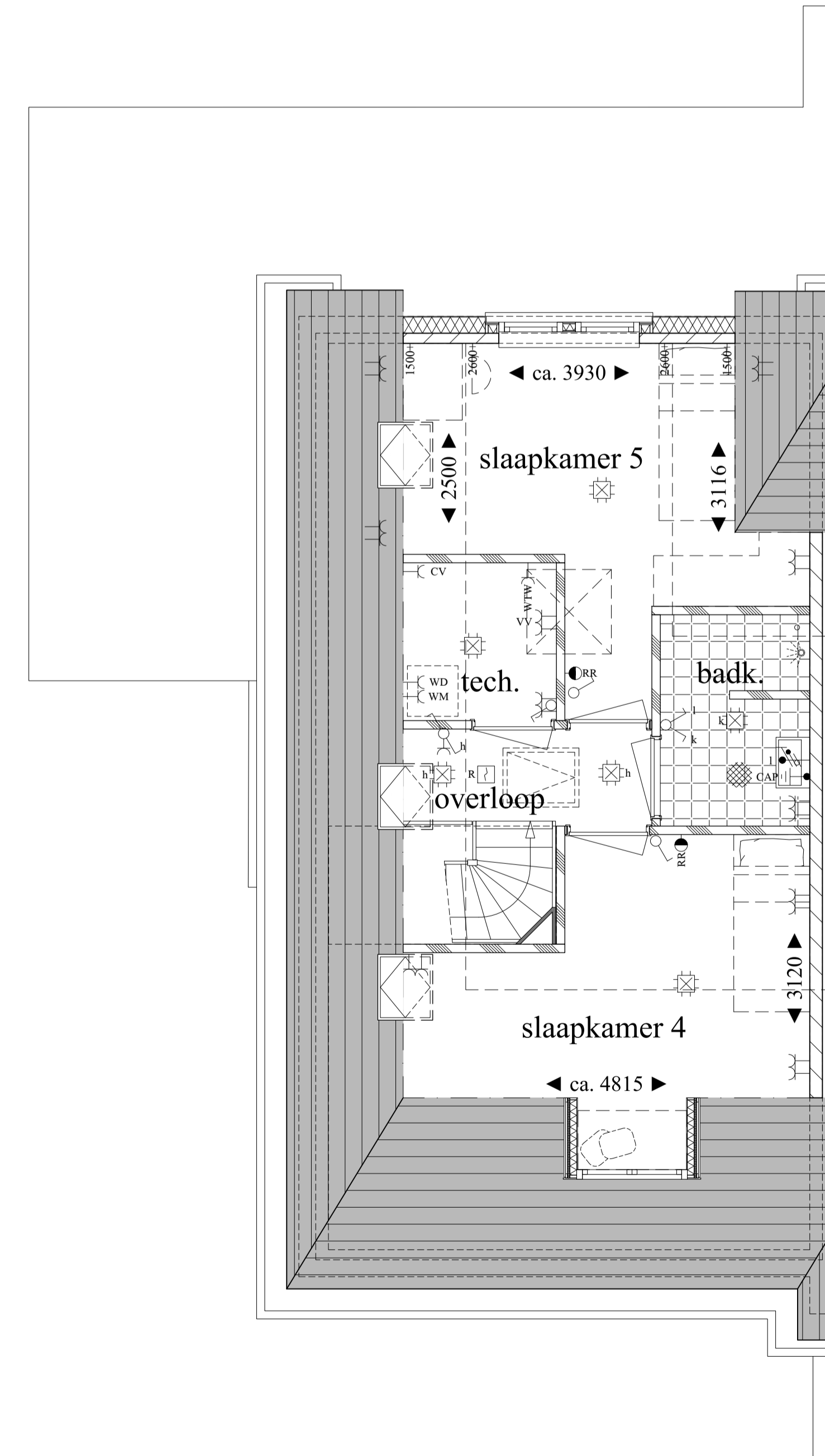
tweede verdieping
