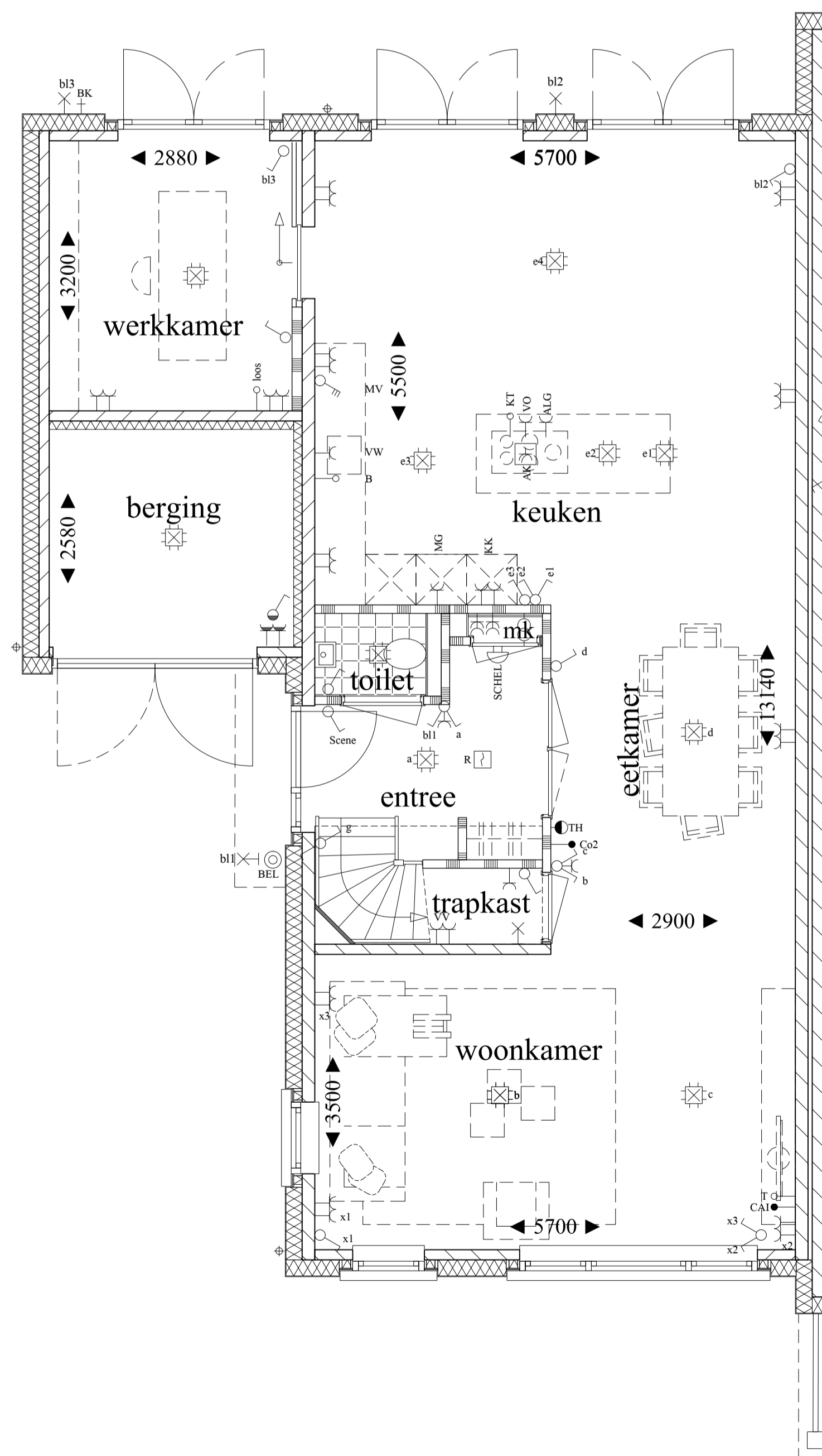
begane grond
