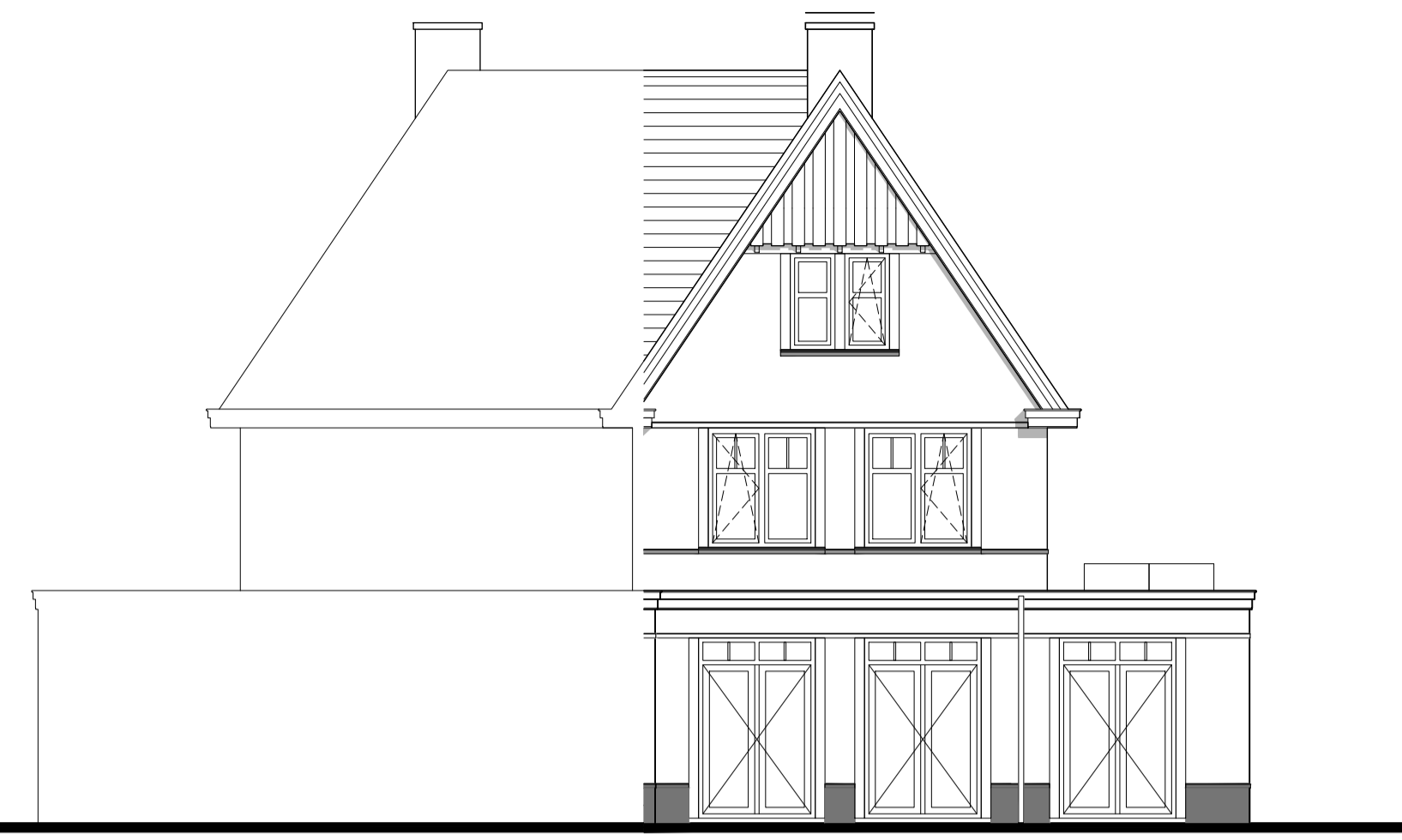
achtergevel
