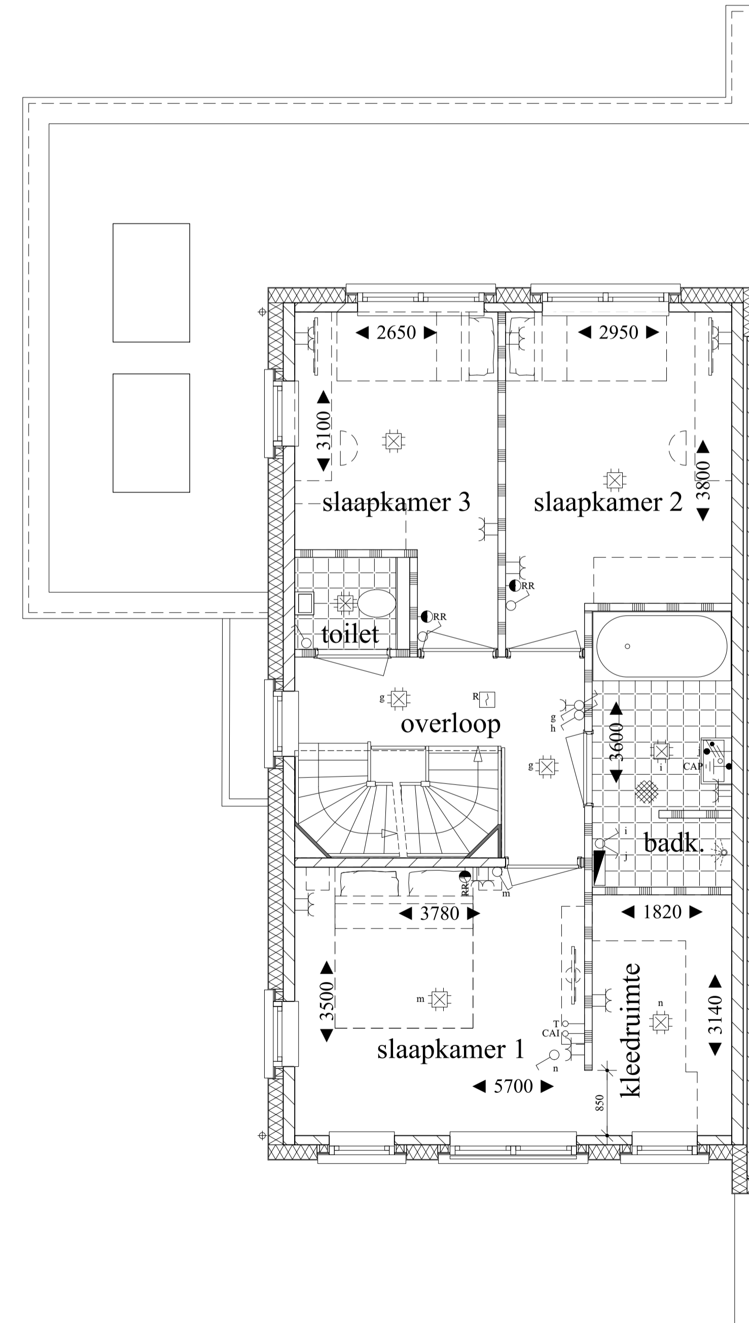
eerste verdieping
