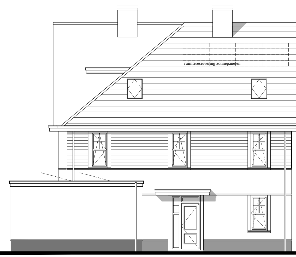
linkerzijgevel
