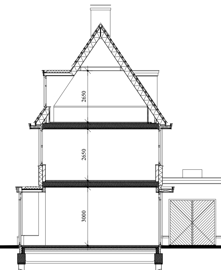
doorsnede
