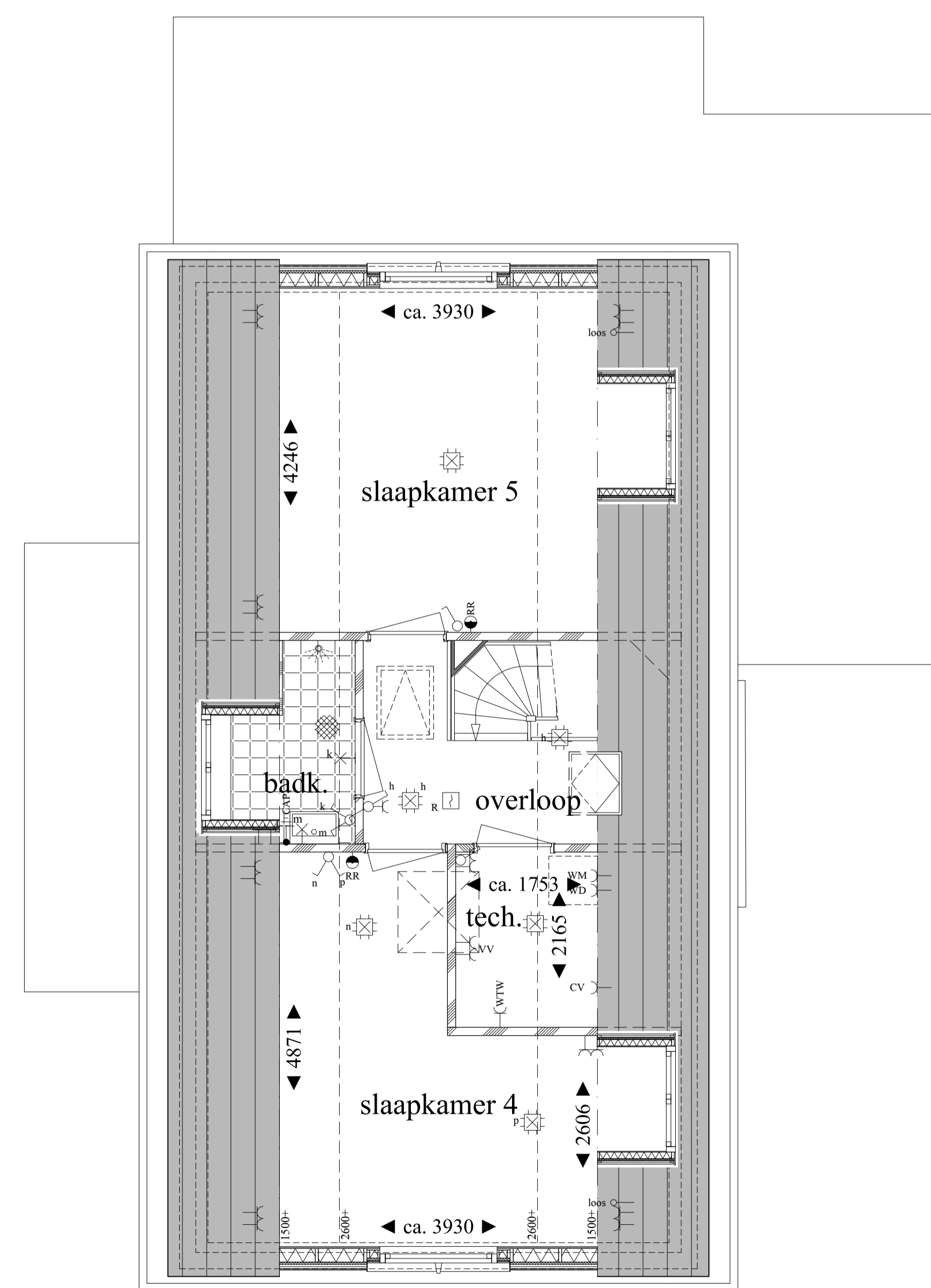
tweede verdieping
