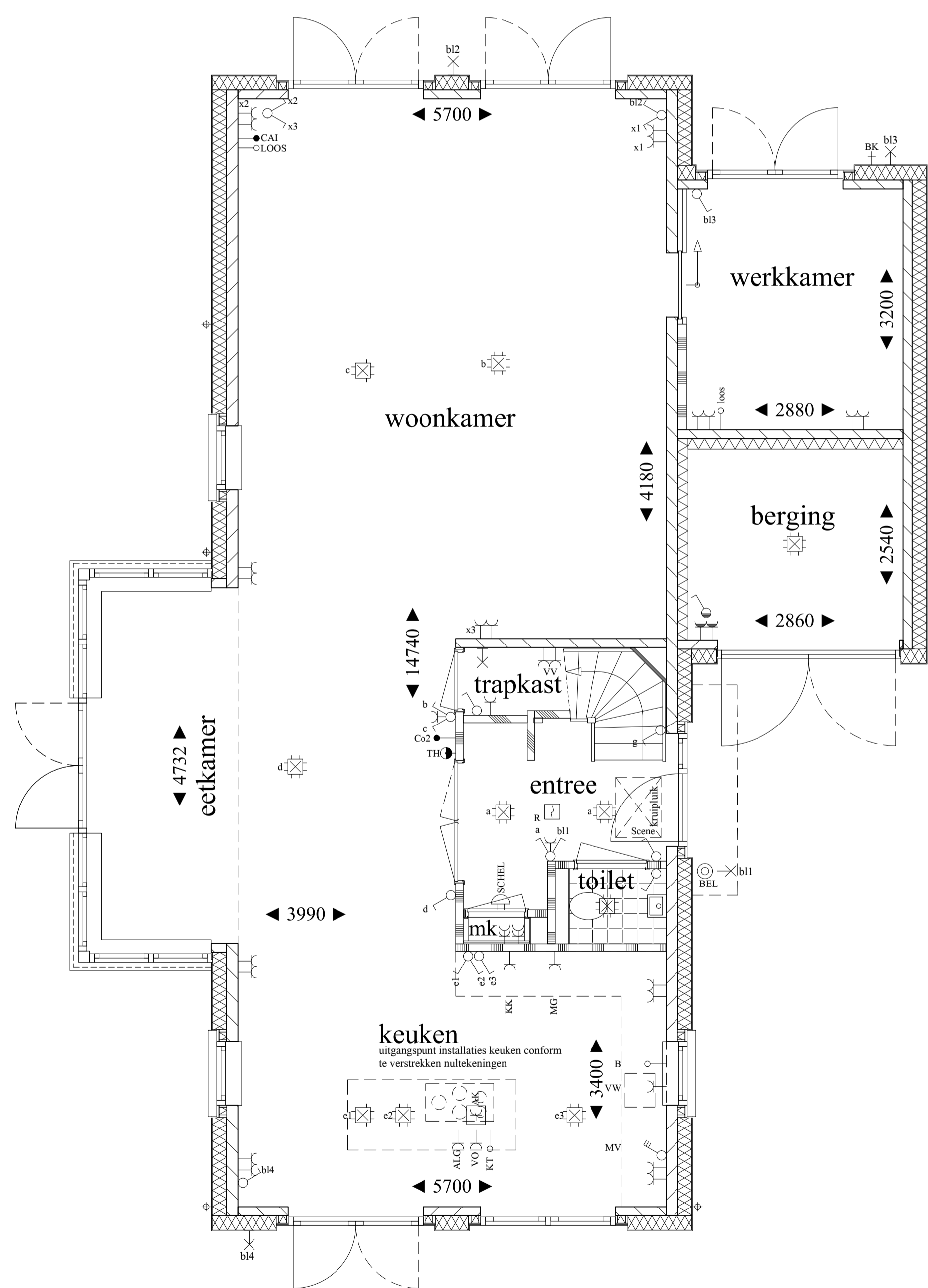
begane grond
