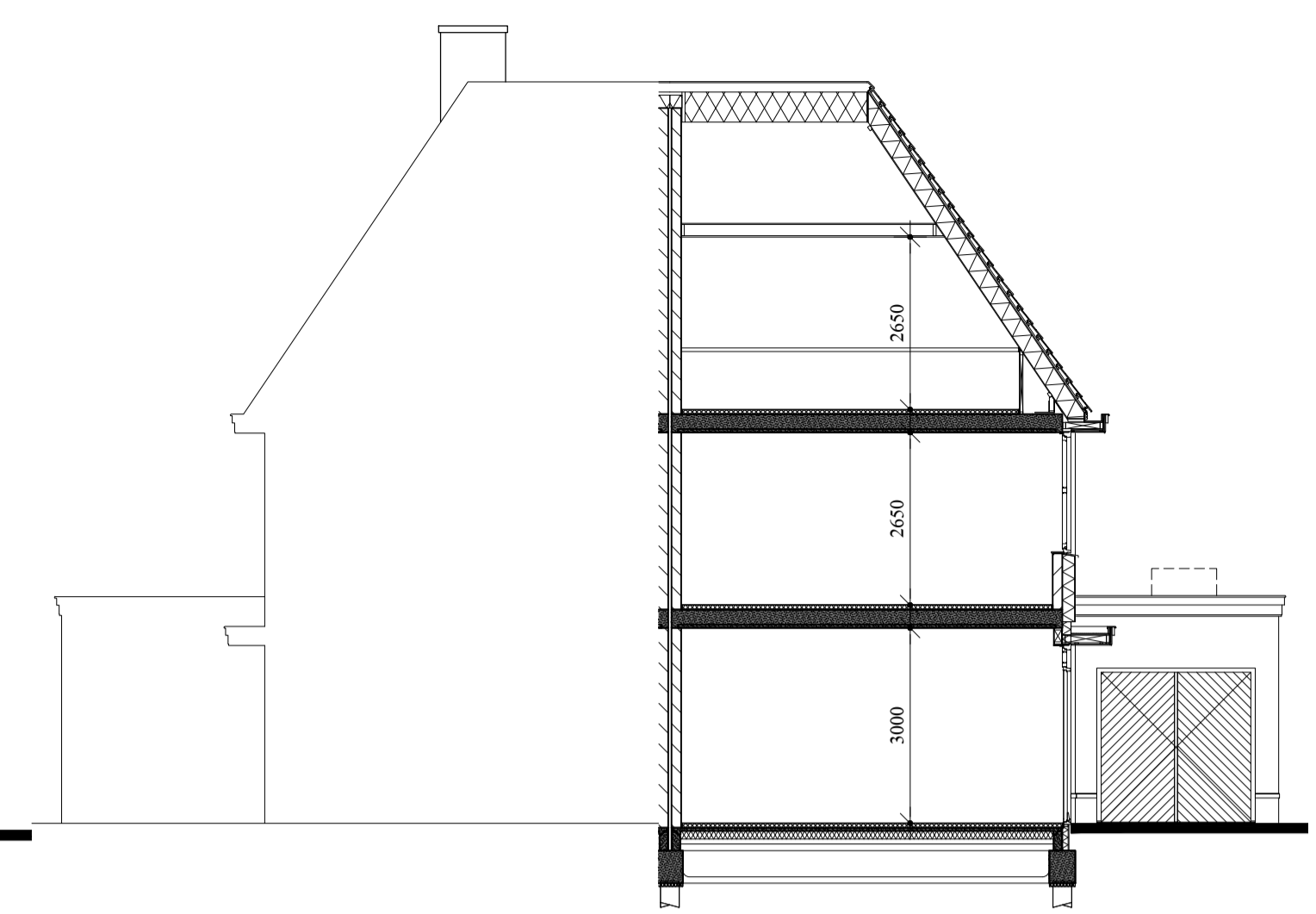
doorsnede
