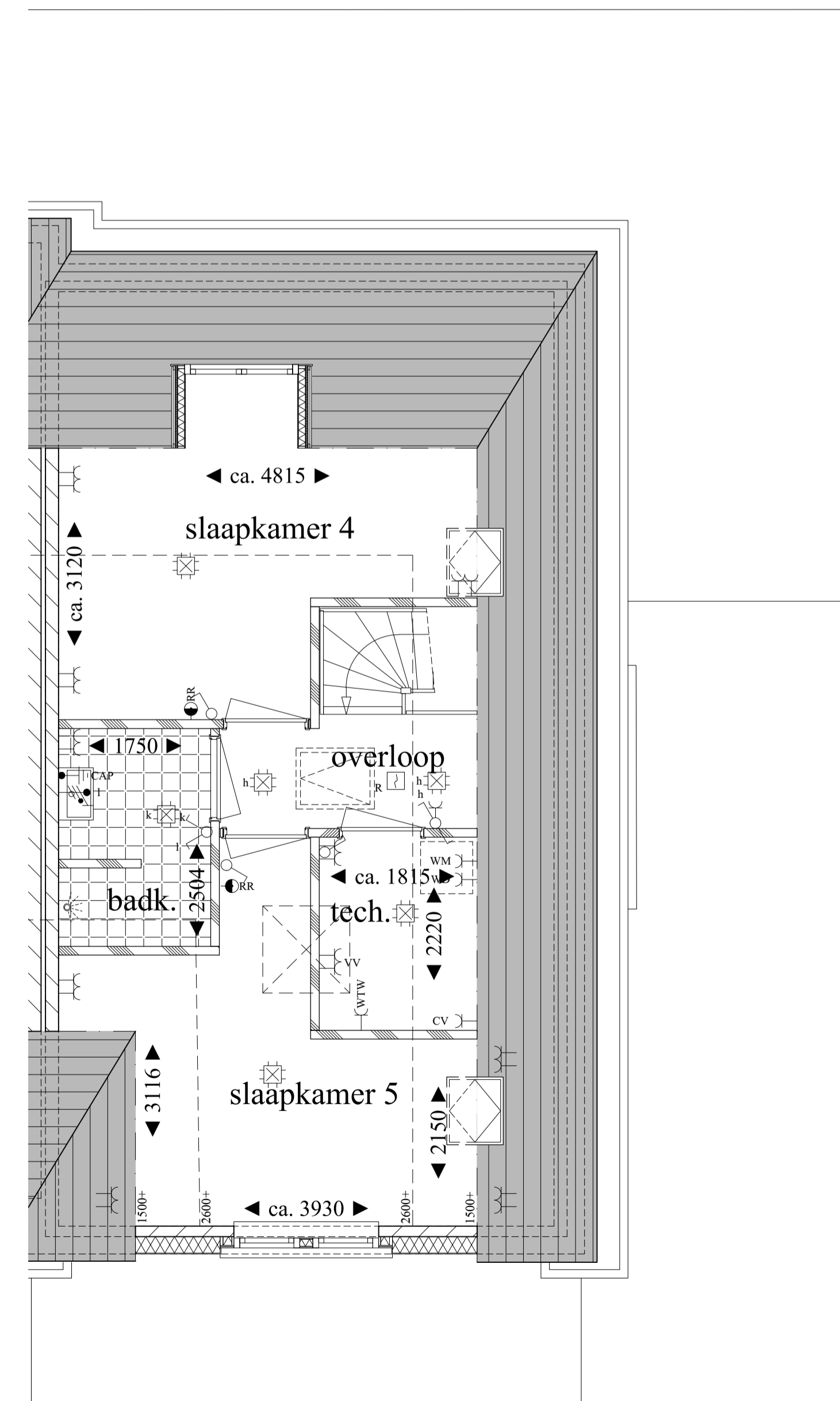
tweede verdieping
