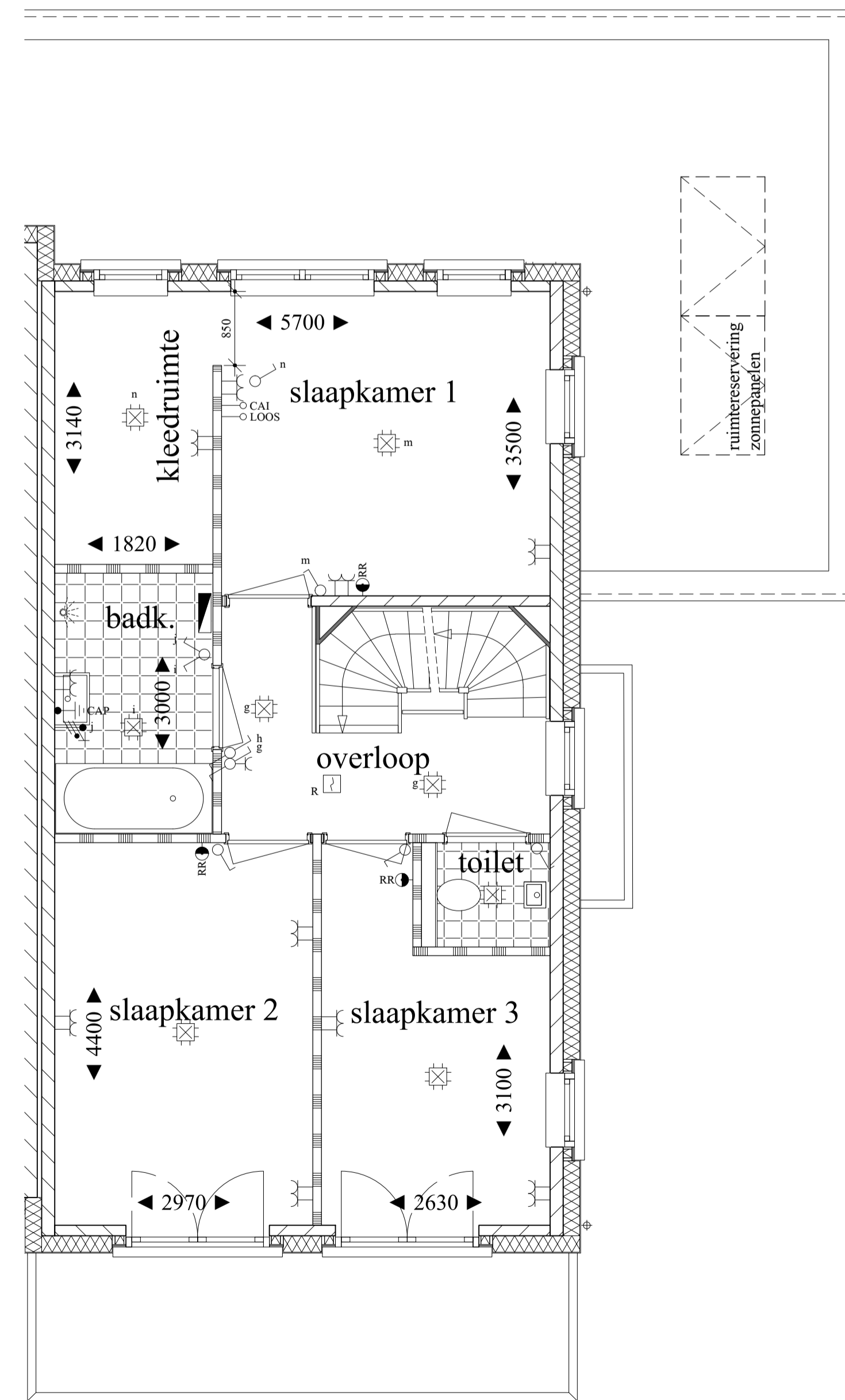
eerste verdieping
