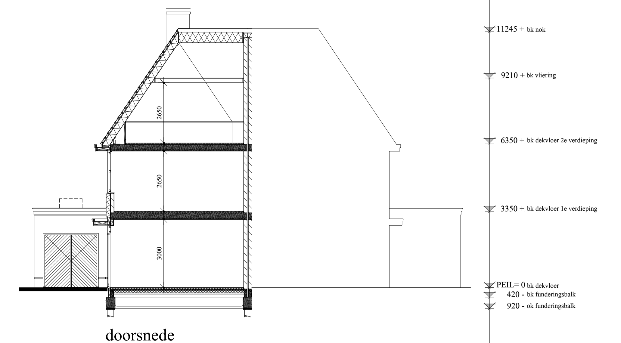
doorsnede
