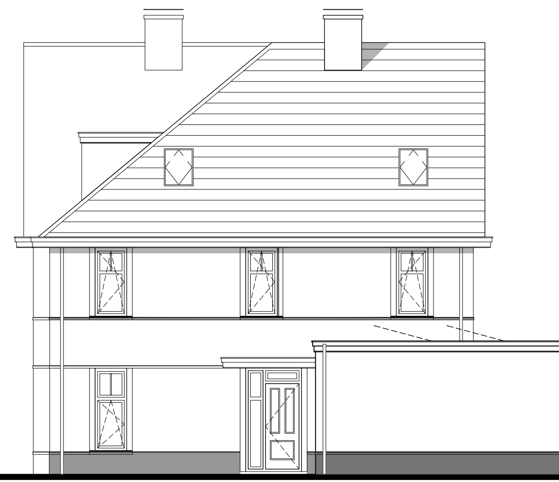
rechterzijgevel
