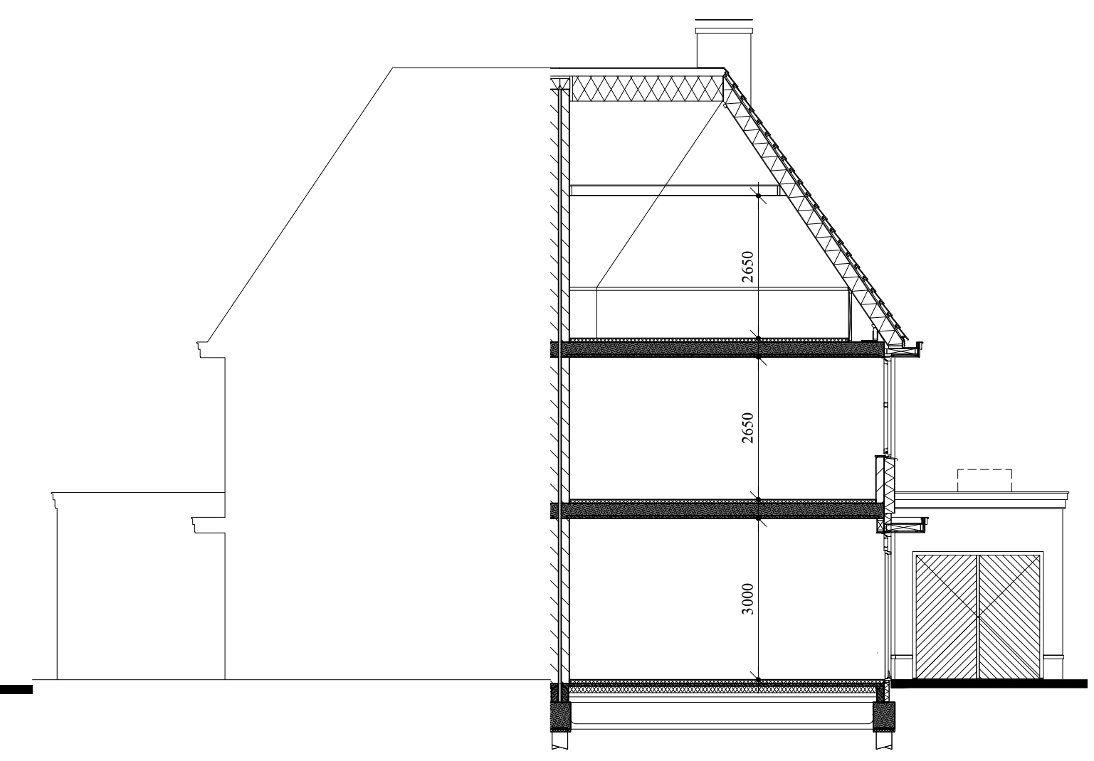
doorsnede
