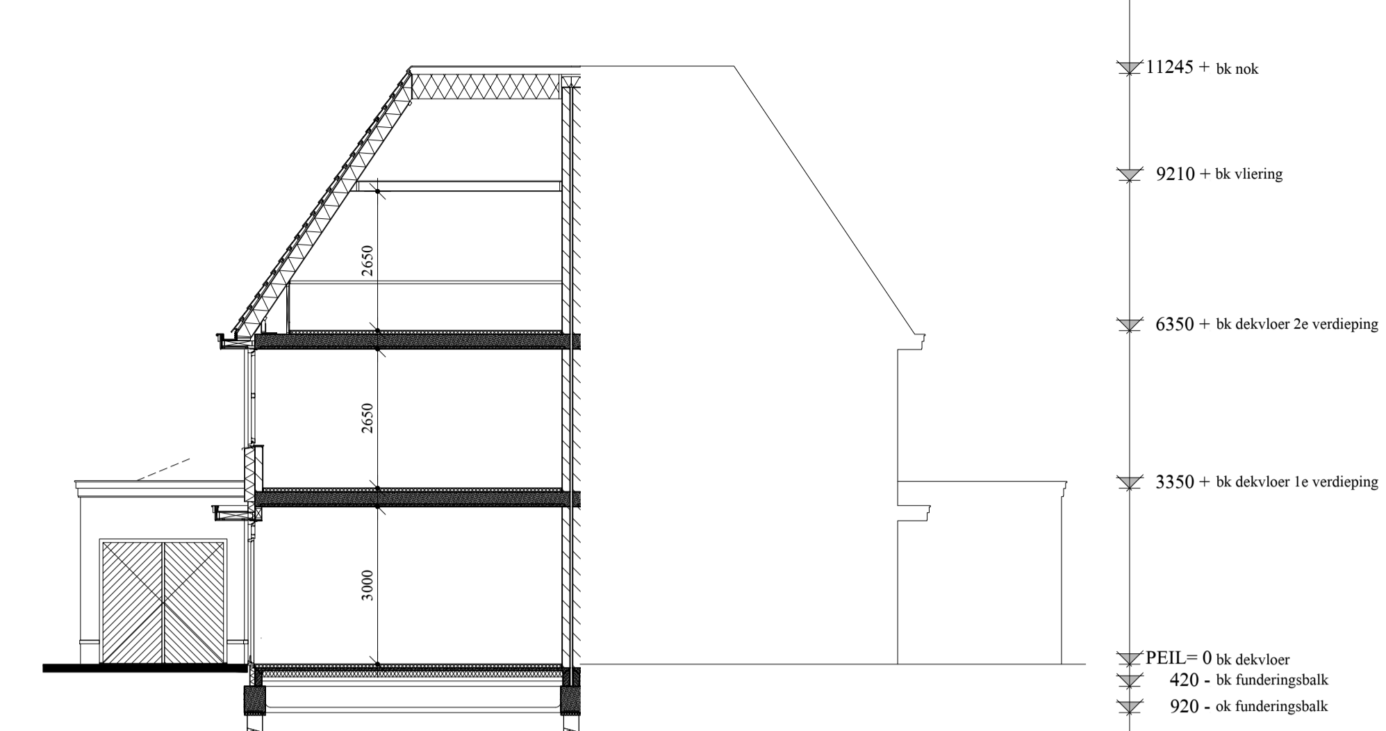
doorsnede
