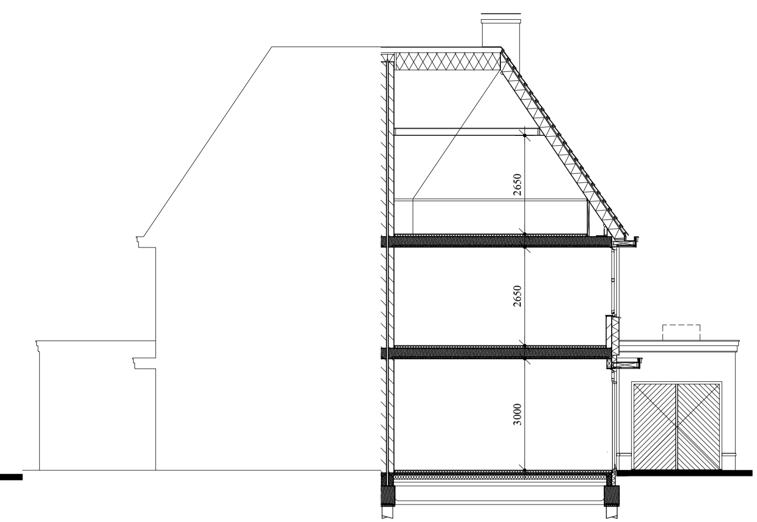
doorsnede
