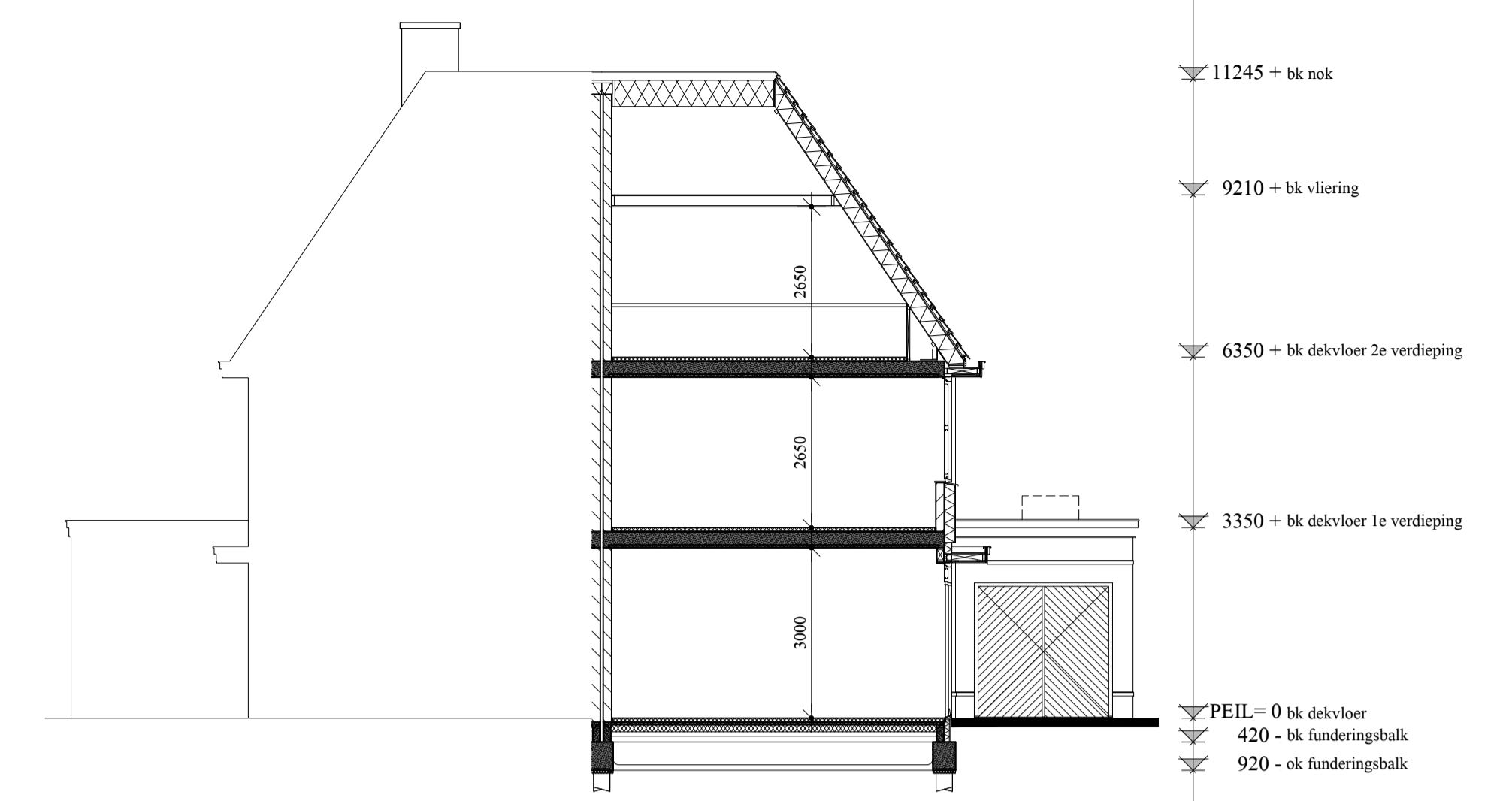
doorsnede
