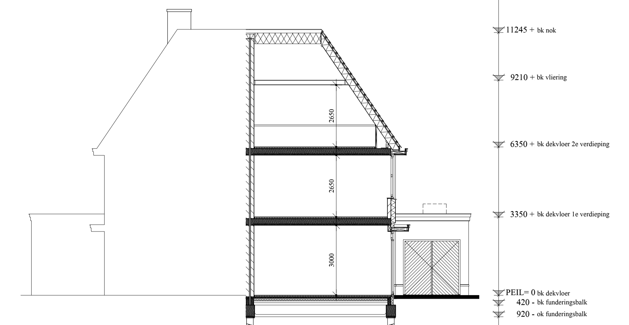
doorsnede
