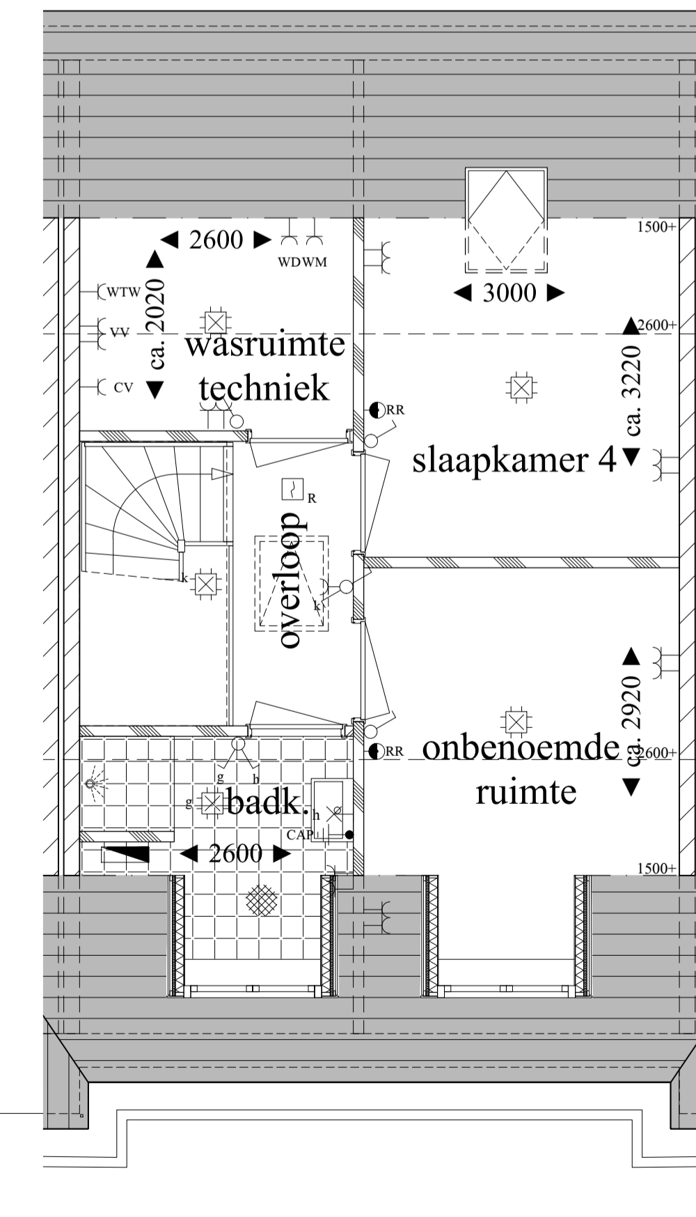
tweede verdieping
