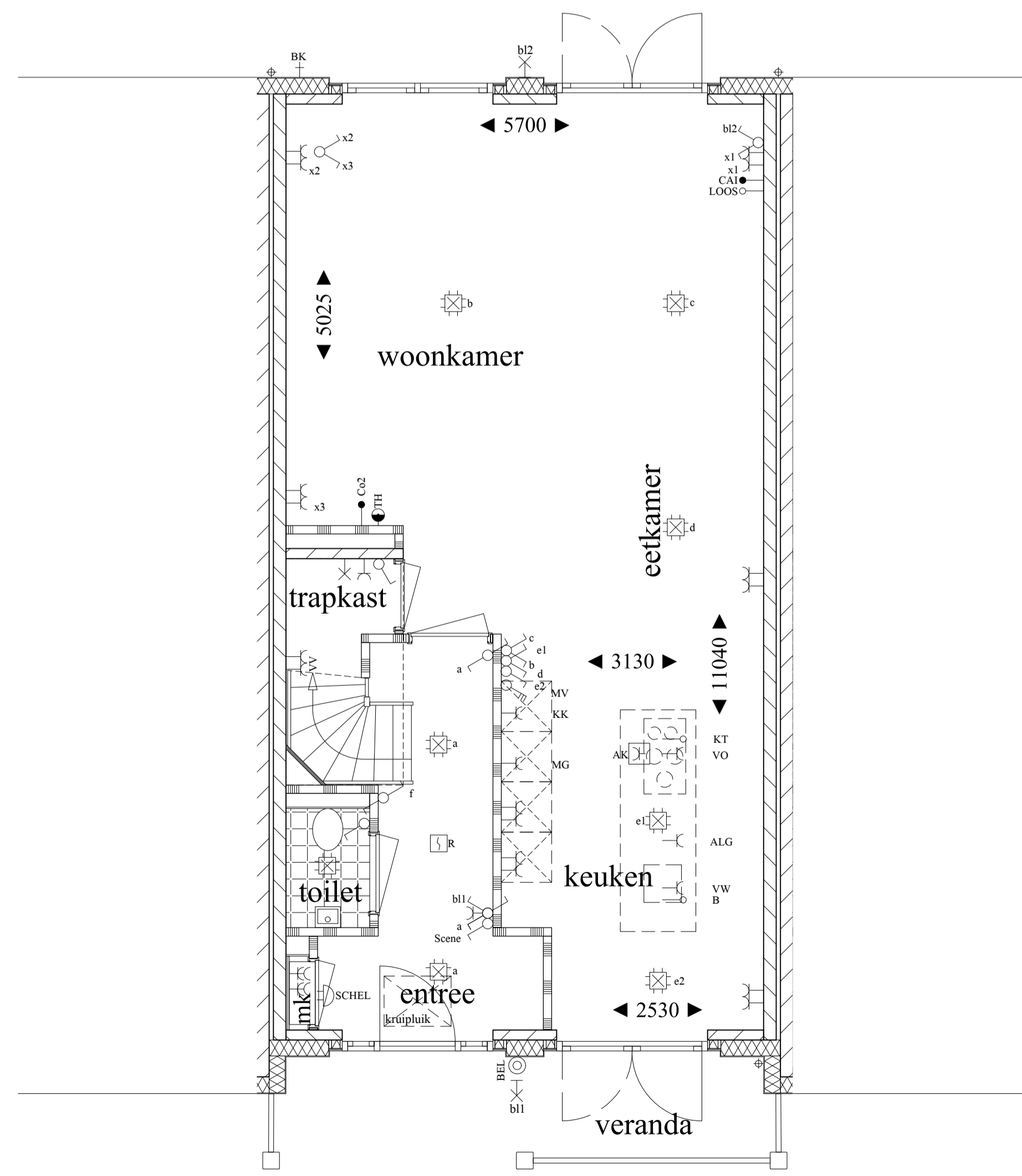
begane grond
