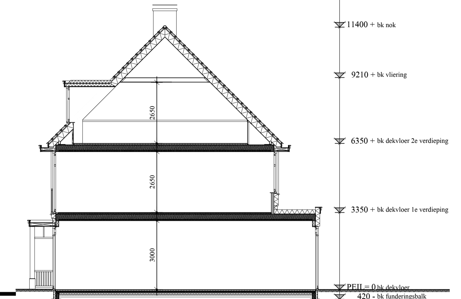
doorsnede
