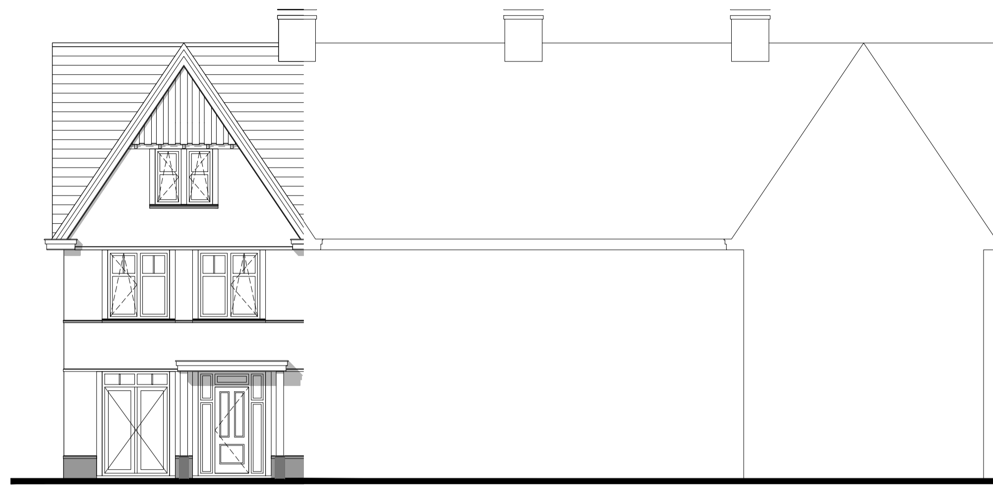
voorgevel
