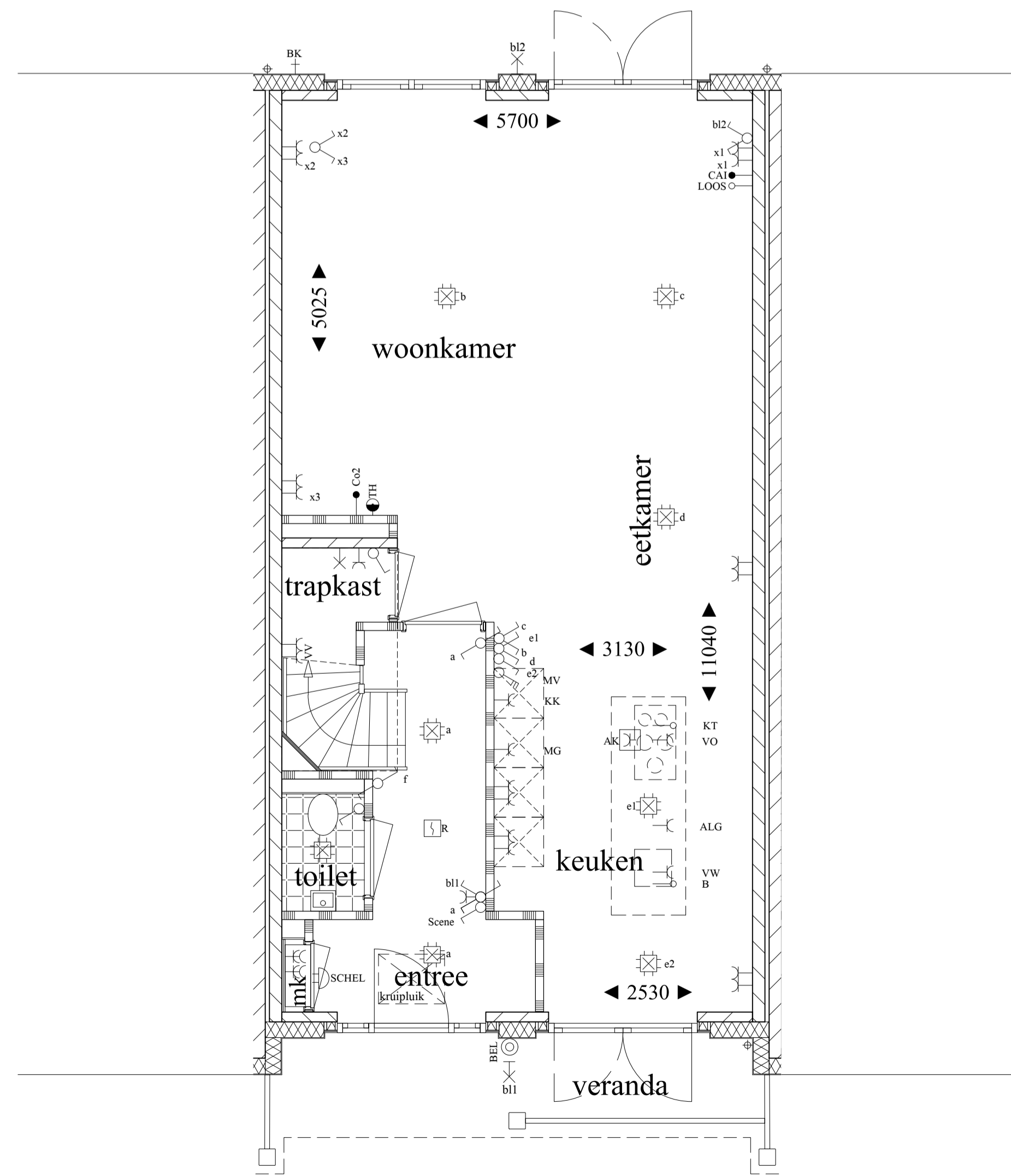
begane grond
