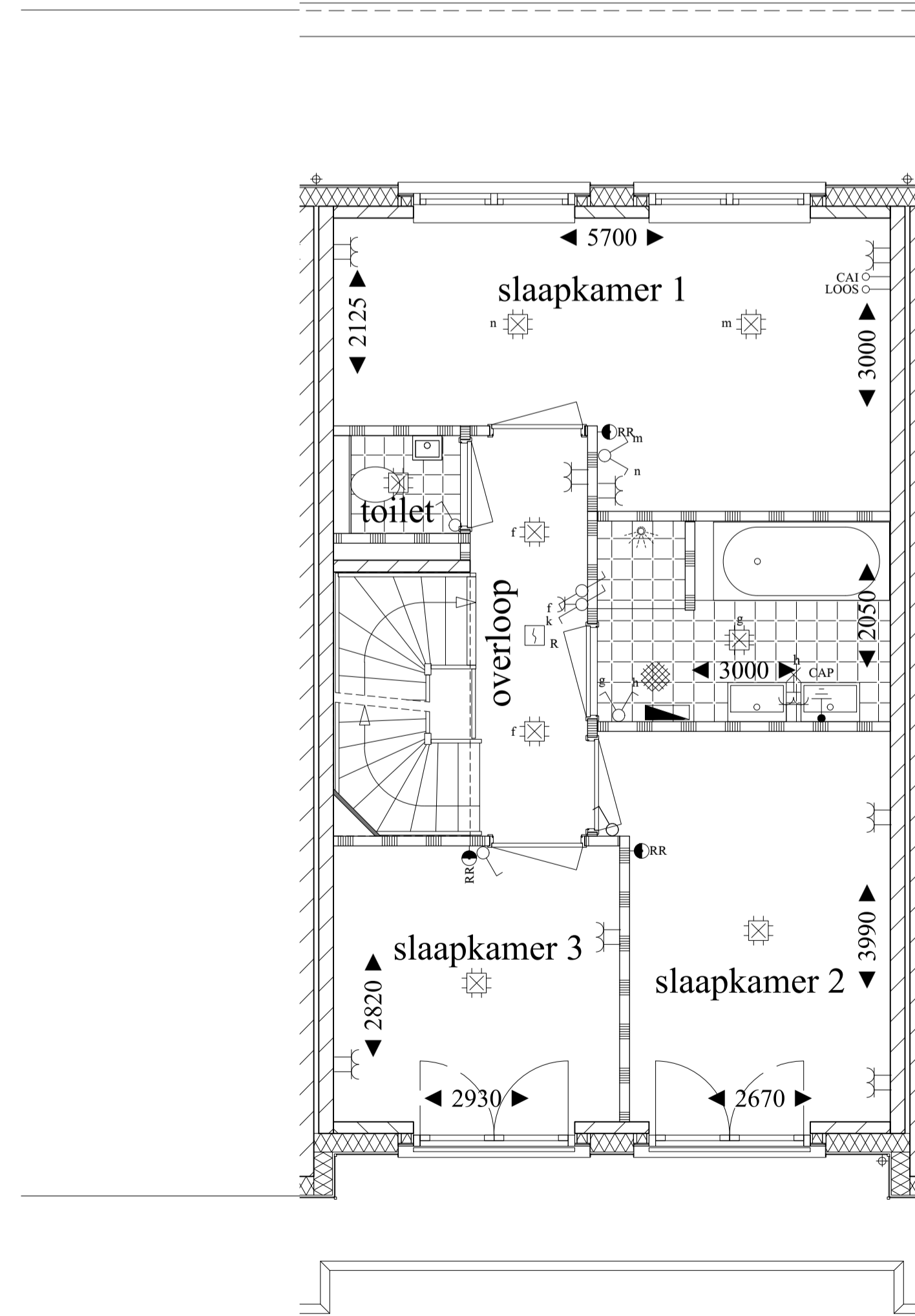
eerste verdieping
