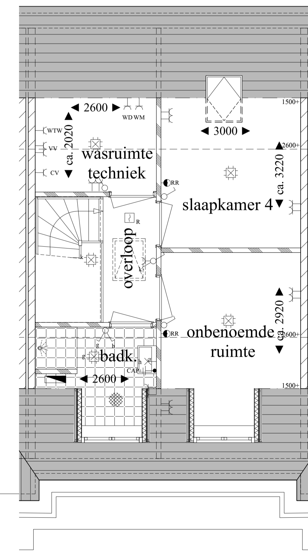
tweede verdieping
