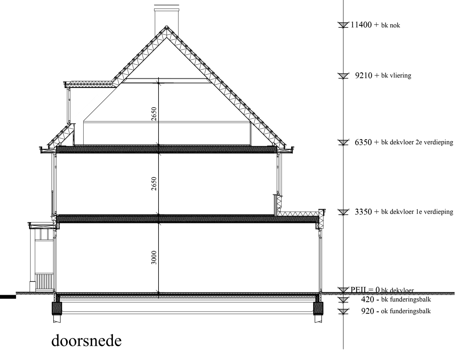
doorsnede
